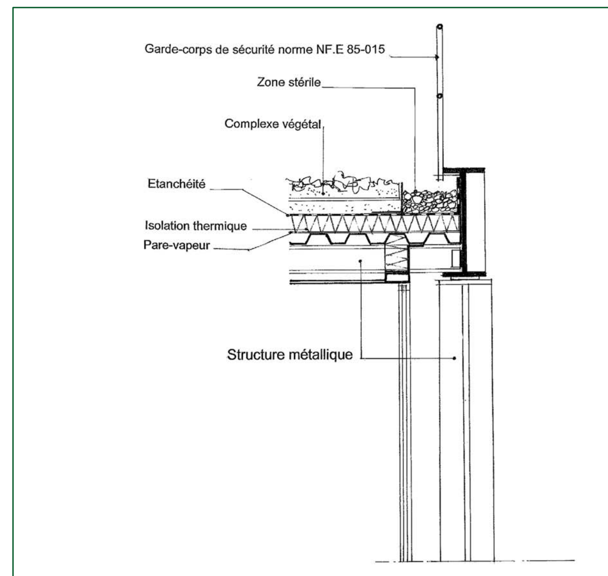
Coupe d'une toiture-terrasse à structure métallique
