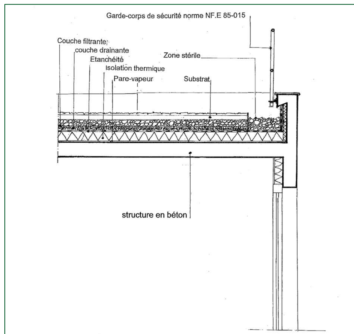
Coupe d'une toiture-terrasse à structure en béton
