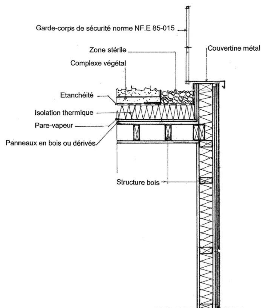
Coupe d'une toiture-terrasse à structure bois
