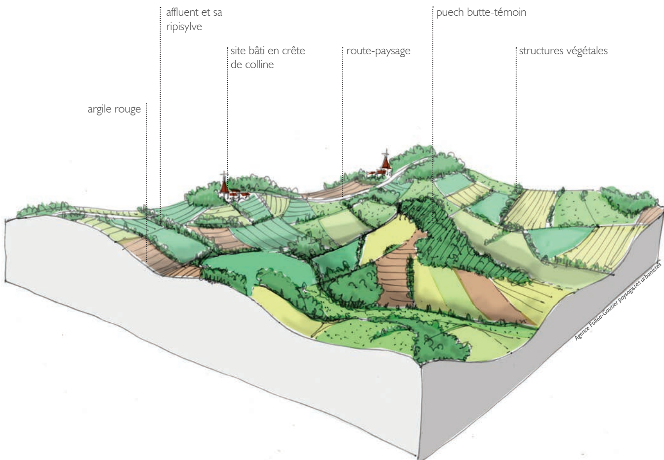
Bloc diagramme des collines de l'albigeois
