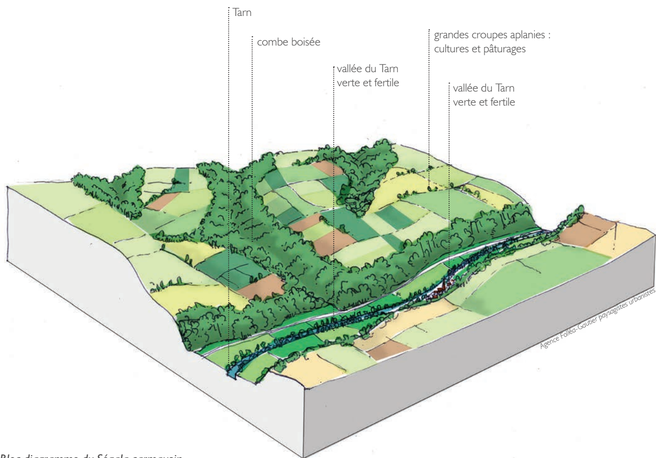
Bloc diagramme du Ségala carmausin
