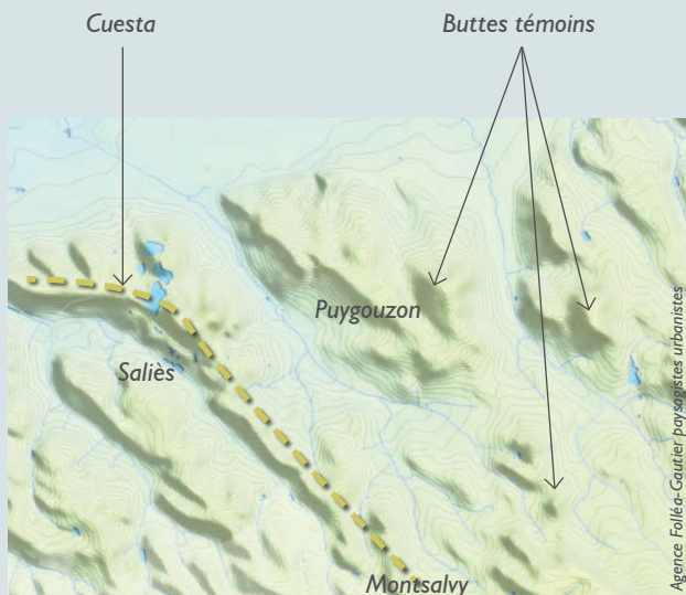
Carte morphologique de la Cuesta et des buttes témoins
