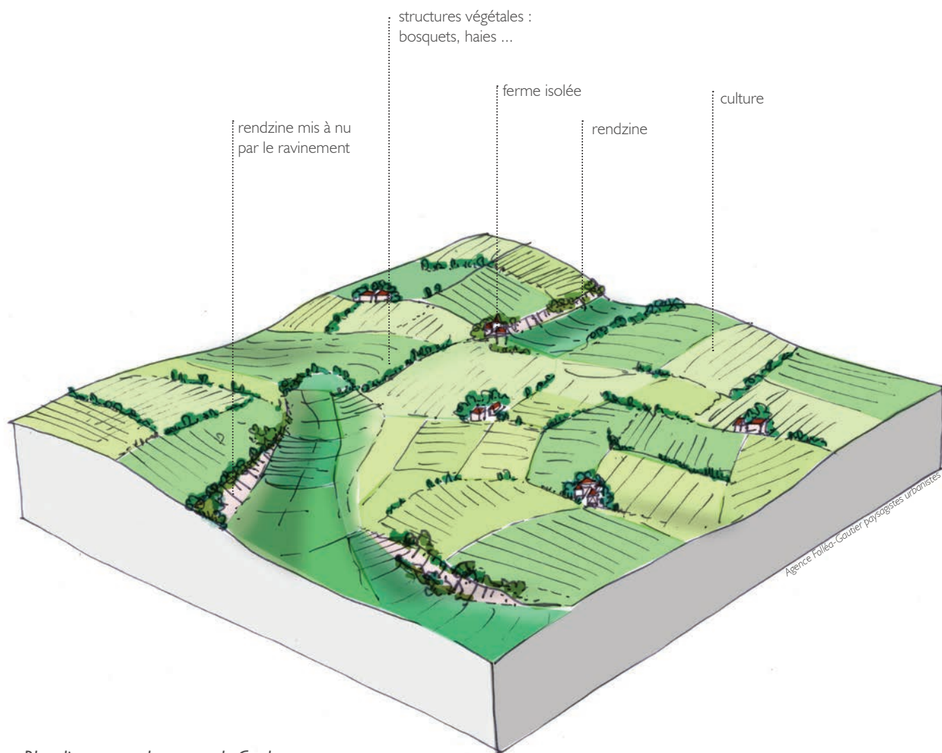
Bloc diagramme du causse de Cordes
