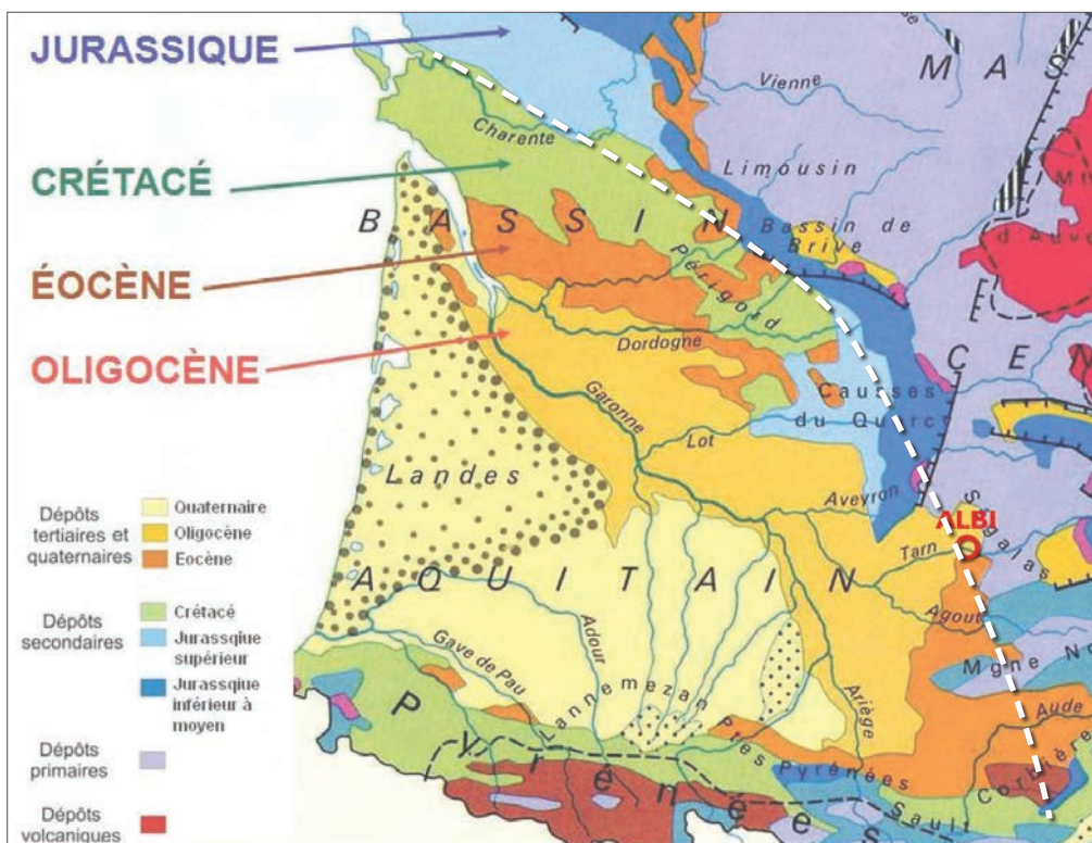
Carte géologique de l'Aquitaine - source : internet
