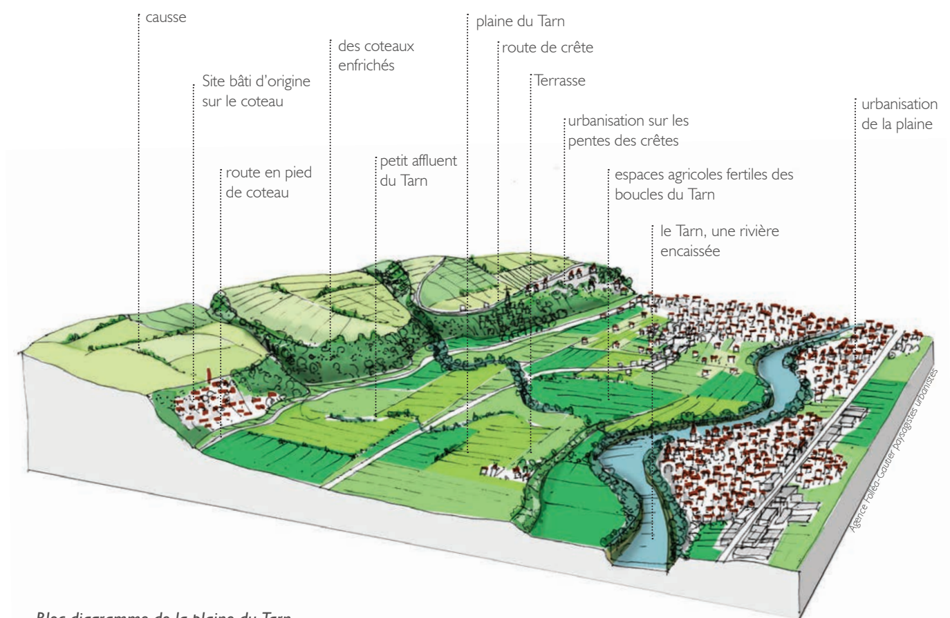
Bloc diagramme de la plaine du Tarn
